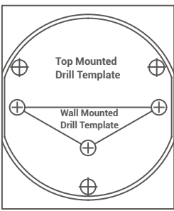
Bohrschablone (×1)
