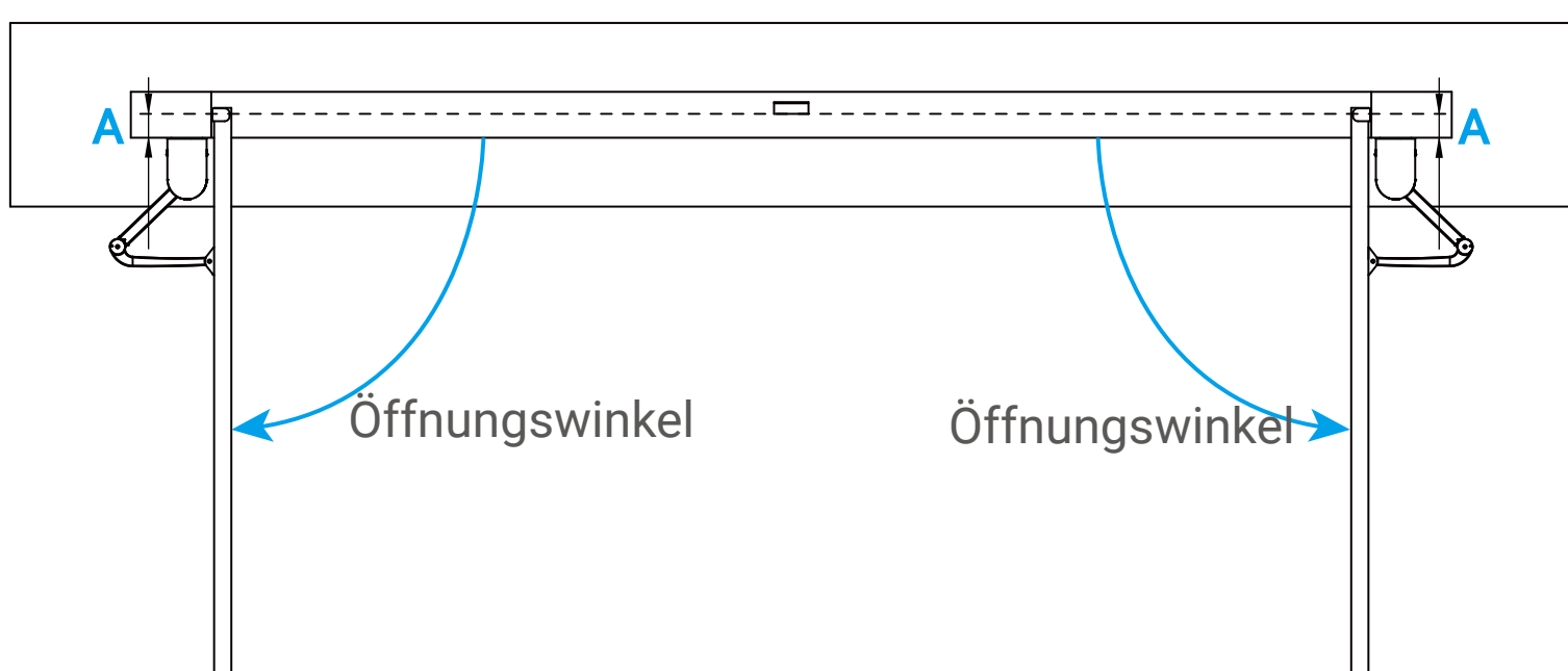
Draufsicht
