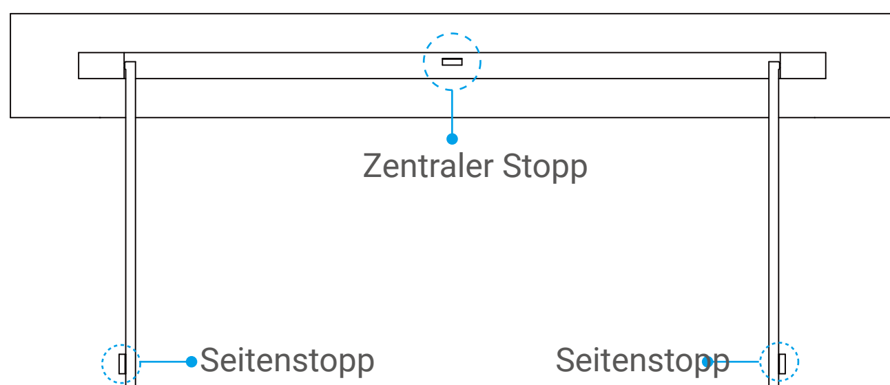
Draufsicht
